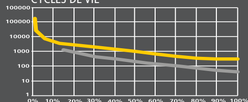
PROFONDEUR DE DÉCHARGE N° DE CYCLES À 50% DE LA CAPACITÉ NOMINALE
